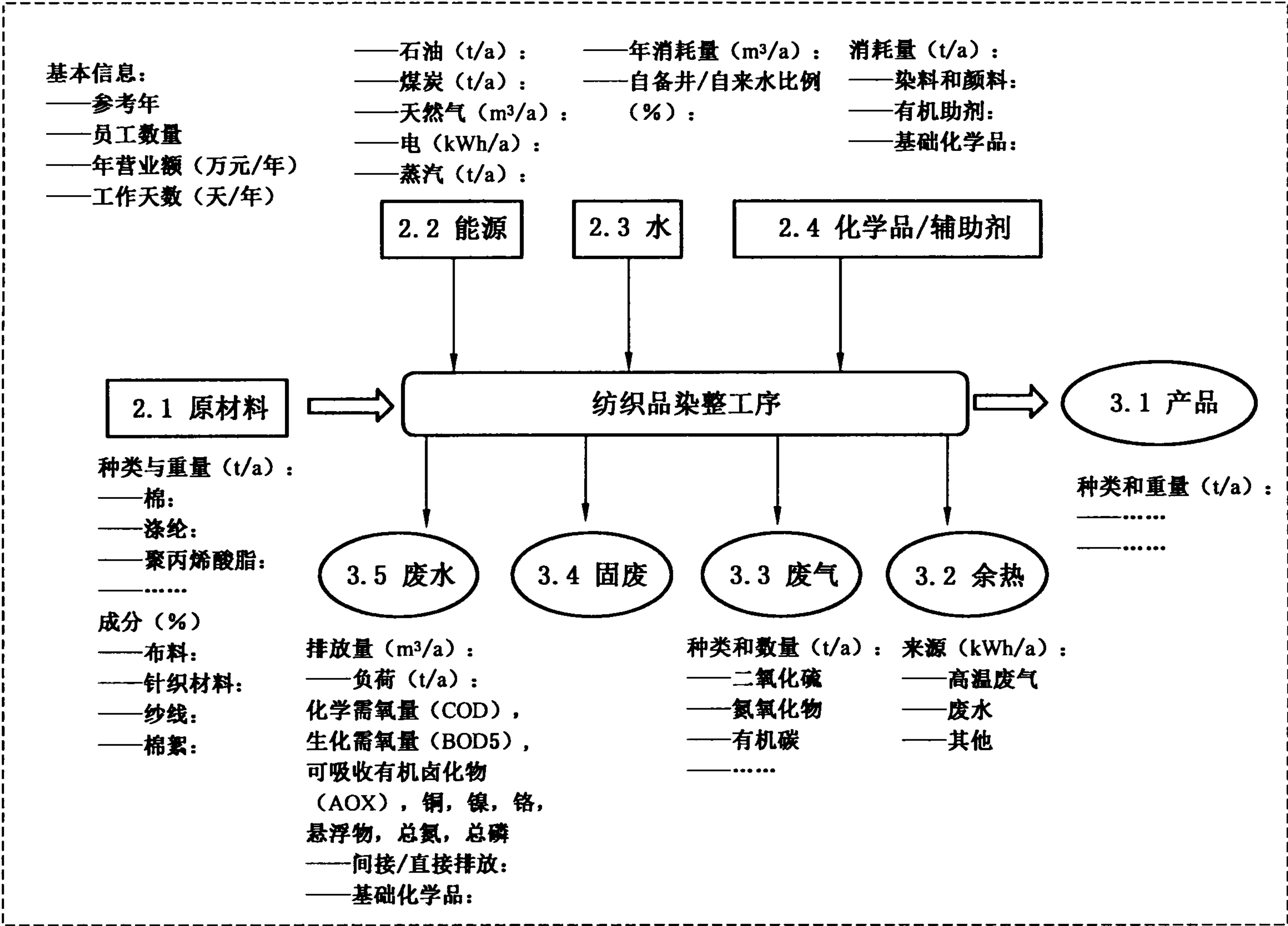
图 C.1 工序图:染整工序
